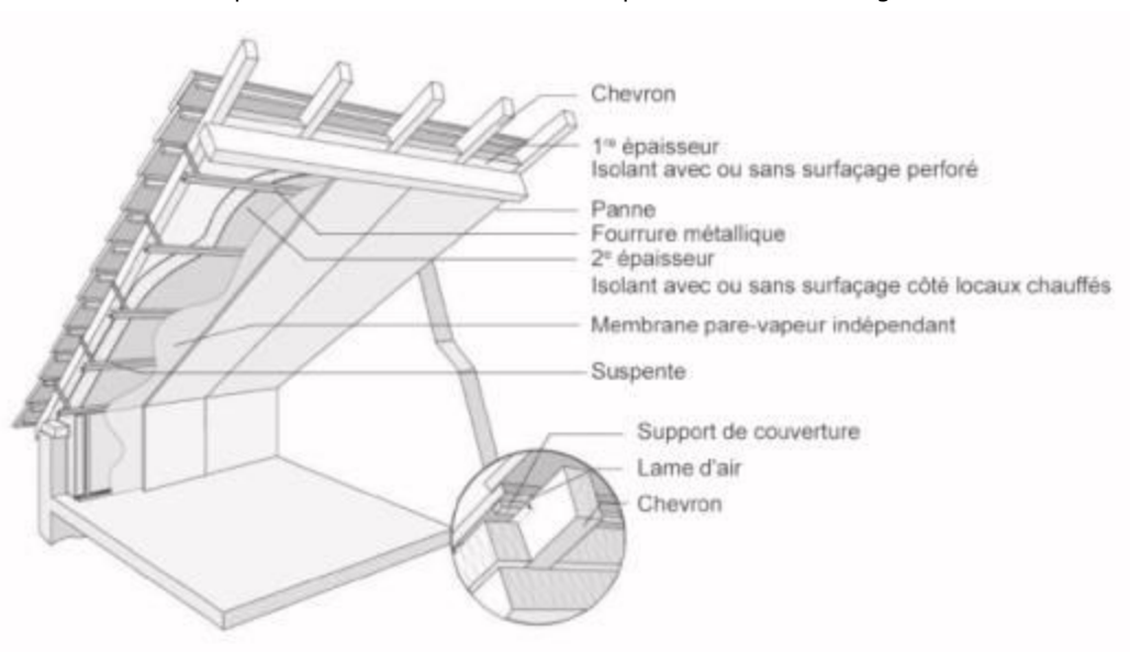
Figure 1- Mise en œuvre des épaisseurs non semi-rigide
